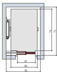
Kabina s jedním vstupem T2 Teleskopické posuvné dveře (2-panelové)
